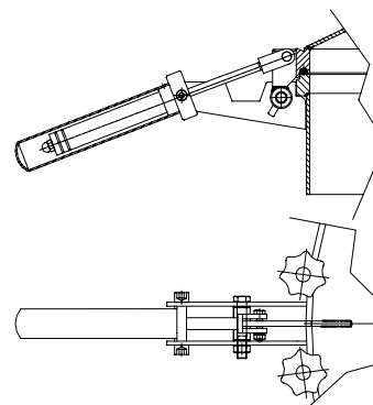
Sistema de molas a gás (versão simples)
