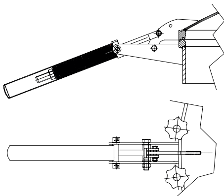
Sistema de molas de disco (versão simples)
