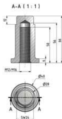
Collar nut M12/M16 Art. No. 2031-A4
