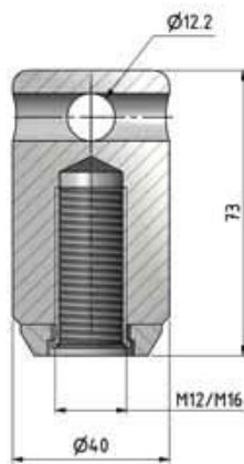
Blind hole nut M12/16 Art. Nr. 2023/ 2024-A4
